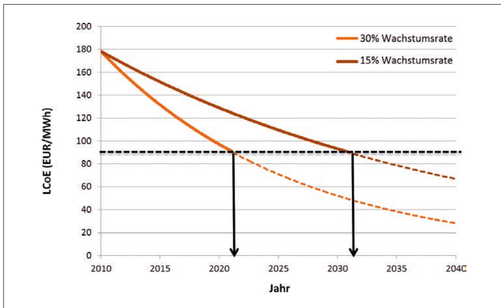
Abb. 4 Entwicklung der LCoE-Kosten ( Lifetime Cost of Electricity ) über Zeit für solarthermische Kraftwerke, die bei 15% (niedrig) und 30% (hoch) Wachstumsraten pro Jahr installiert wurden (basierend auf einer Lernrate von 15%).
