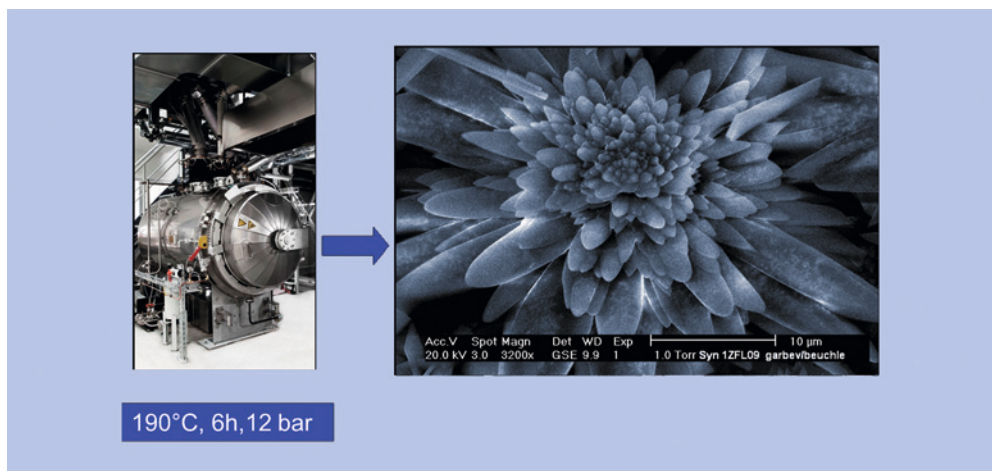
Abb. 6 Technisches Verfahren zur Herstellung von hydraulisch aktivem Calciumhydro-silikat („Celitement“): Entsäuertes Rohmehl wird gemeinsam mit Wasser in einem Autoklaven ( links ) zu z. B. \alpha\text{-Ca}_2(\text{SiO}_4\text{H})(\text{OH}) ( rechts ) umgesetzt.
