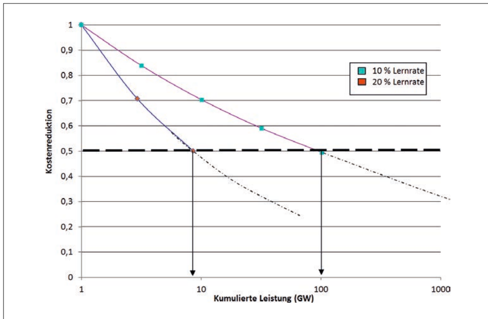
Abb. 3 Relative Kosten der CSP-Technologie als Funktion der kumulierten installierten Leistung für eine Lernrate von 10 und 20%.
