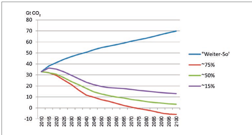
Abb. 3 Die Herausforderung des ambitionierten Klimaschutzes. Projektionen der globalen Emissionen bei einem energiepolitischen ‚Weiter-So‘ gegenüber drei Reduktionspfaden, die das 2 °C-Ziel mit unterschiedlichen Wahrscheinlichkeiten erreichen. Die Differenz zwischen der ‚Weiter-So‘-Entwicklung und den Reduktionspfaden zeigt die ‚Vermeidungslücke‘. (Quelle: EDENHOFER et al. 2010a, S. 23)
