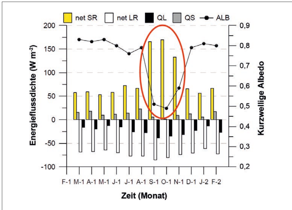
Abb. 3 Monatsmittel der Energieflüsse an der Automatischen Wetterstation 1 am Nördlichen Eisfeld des Kilimandscharo zwischen Februar 2001 und Februar 2002: absorbierte Sonnenstrahlung (gelb), Budget der langwelligeren terrestrischen Strahlung (weiß), turbulenter latenter (schwarz) und fühlbarer (grau) Wärmestrom. Die mittlere monatliche Albedo (schwarze Linie) ist das Verhältnis von reflektierter zu einfallender kurzwelliger Sonnenstrahlung und bezieht sich auf die rechte y-Achse. Die Ellipse markiert eine im Text angesprochene Periode im Jahr 2001. Datenquelle: MÖLG und HARDY 2004.
